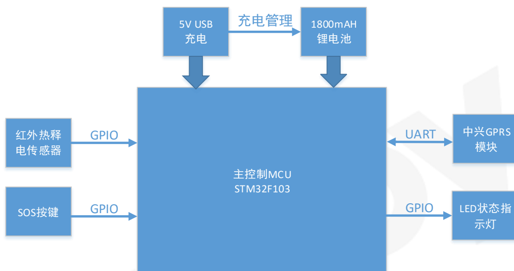
图 1 硬件功能框图
